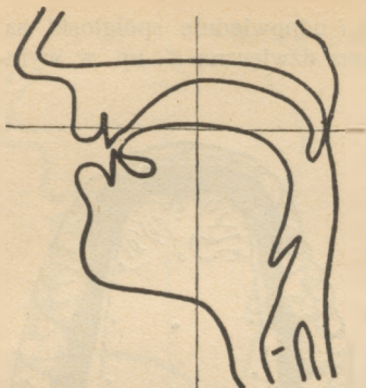
Rys. 29. Nastawy spółgłoski s.
