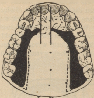
Rys. 43. Miejsce zetknięcia przy ż (plama czarna) i ś (jeszcze po linię kreskowaną).
