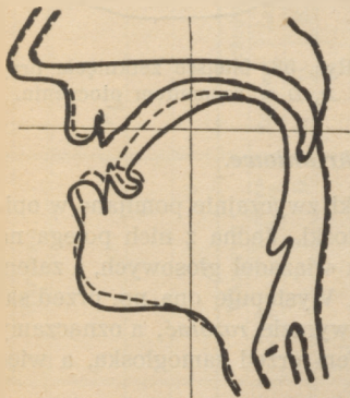
Rys. 55. Nastawy spółgłosek \chi (linia ciągła) i \check{\chi} (linia przerywana).
