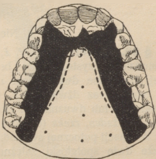
Rys. 39. Miejsce zetknięcia przy ż (czarna plama) i ć (jeszcze po linię kreskowaną).
