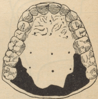
Rys. 54. Miejsce zetknięcia przy k w wyrazie kamień .
