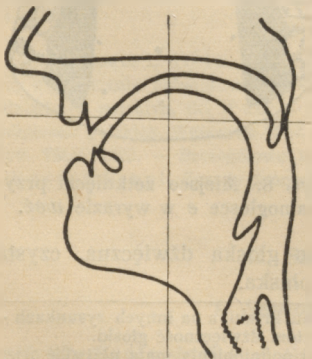
Rys. 11. Nastawy samogłoski i .
