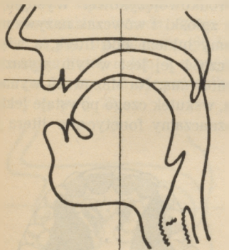
Rys. 7. Nastawy samogłoski e .
