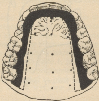
Rys. 28. Miejsce zetknięcia przy spółgłoskach: d , n (miejscie zaczerńnione) i t (to samo miejsce szersze do linii przerywanej). 1
