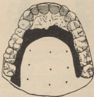
Rys. 49. Miejsce zetknięcia przy l w wyrazie las .
