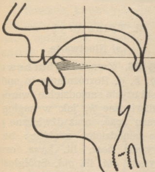
Rys. 48. Nastawy spółgłoski l .
