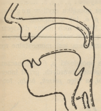
Rys. 19. Połączony obraz nastaw samogłosek ą i a.
