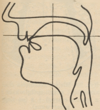
Rys. 27. Nastawy spółgłoski t .
