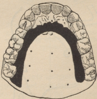
Rys. 51. Miejsce zetknięcia przy l' w wyrazach len , lis . 1
