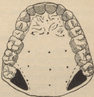
Rys. 56. Miejsce zetknięcia przy \chi w wyrazie ach (plama czarna) i w wyrazie hak (do linji przerywanej).
