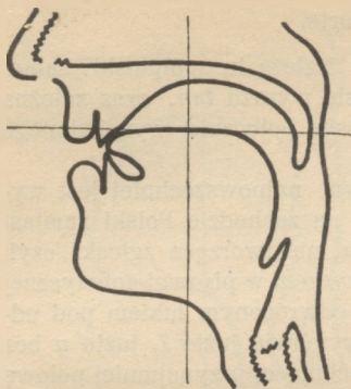
Rys. 35. Nastawy spółgłoski n .
