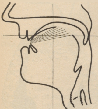
Rys. 50. Nastawy spółgłoski l' .
