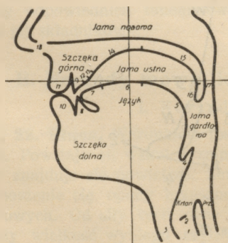
Rys. 4. Obraz narządów mowy w czasie oddychania. 1
