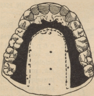
Rys. 44. Miejsce zetknięcia przy d (czarna plama) i t (jeszcze po linię przerywaną).
