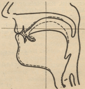
Rys. 25. Nastawy spółgłosek m (linje ciągłe) i m̃ (linje przerywane).
