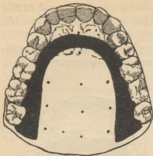
Rys. 52. Miejsce zetknięcia przy ŋ w wyrazie pączek .
