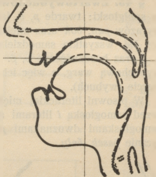
Rys. 20. Połączony obraz nastaw samogłosek ę i e.
