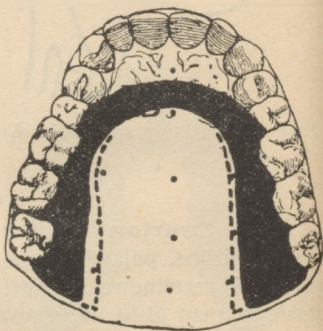
Rys. 46. Miejsce zetknięcia przy ž (plama czarna) i č (jeszcze po linię przerywaną).
