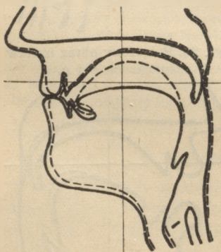
Rys. 23. Nastawy spółgłosek p (linje ciągłe) i p̣ (linje przerywane).
