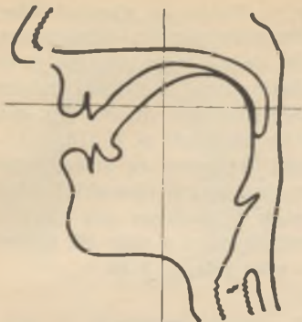
Rys. 57. Nastawy spółgłoski n .
