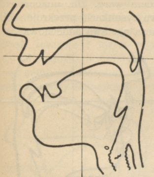
Rys. 13. Nastawy samogłoski o.
