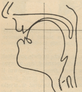
Rys. 40. Nastawy spółgłoski ń .
