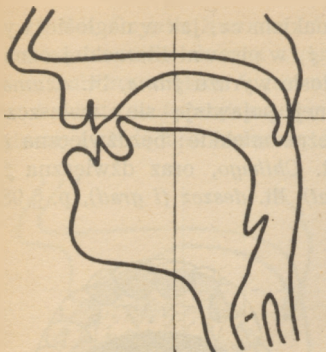
Rys. 42. Nastawy spółgłoski ś.
