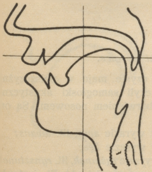
Rys. 15. Nastawy samogłoski u.
