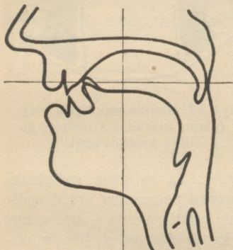
Rys. 45. Nastawy spółgłoski č .
