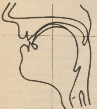
Rys. 38. Nastawy spółgłoski ć.
