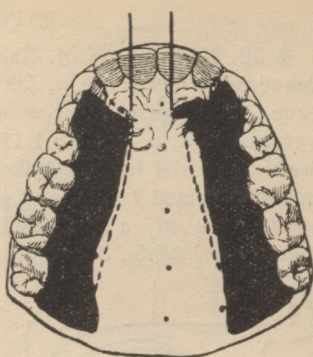
Rys. 37. Miejsce zetknięcia przy ż (czarna plama) i ś (jeszcze po linię kreskowaną).
