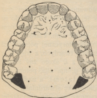
Rys. 59. Samogłoska a w wyrazie pan .
