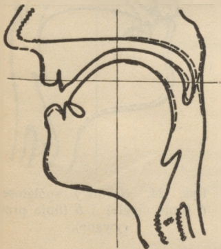
Rys. 21. Połączony obraz nastaw samogłosek i i ɨ.
