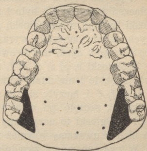
Rys. 60. Samogłoska a w wyrazie śaś .
