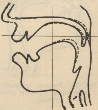
Rys. 22. Połączony obraz nastaw samogłosek o i ɔ.
