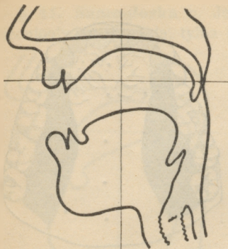
Rys. 5. Nastawy samogłoski a . 1
