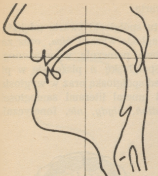
Rys. 36. Nastawy spółgłoski ś.
