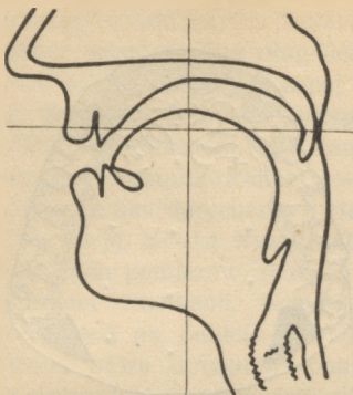
Rys. 9. Nastawy samogłoski y .
