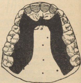
Rys. 41. Miejsce zetknięcia przy ń w wyrazie Mania .
