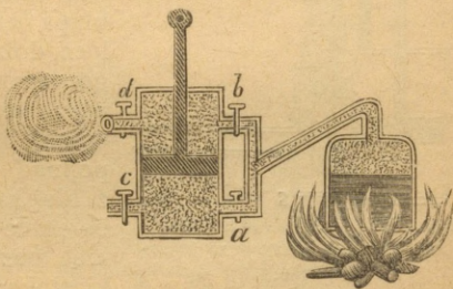
Rys. 57. Kocioł i cylinder z tłokiem oraz rurą, prowadzącą parę pod tłok i nad tłok.
