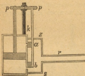
Rys. 58. Drażek otwierający i zamykający kłapy w cylindrze.
