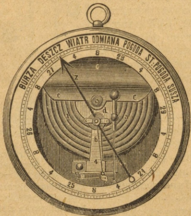
Rys. 63. Barometr metaliczny (aneroid).
