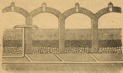
Rys. 51. Wielkie filtry miejskie
