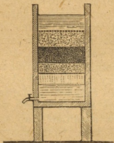
Rys. 50. Filtr domowy.
