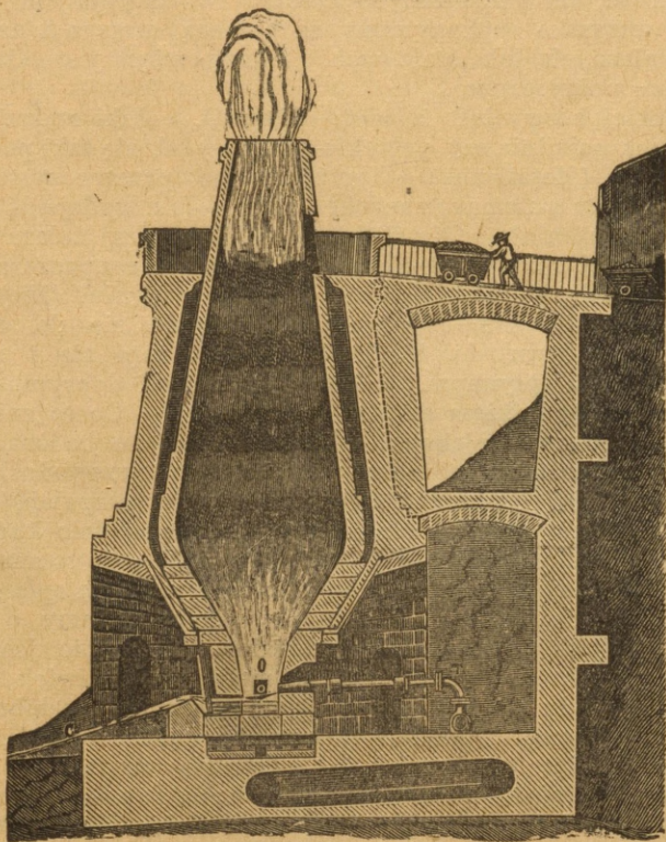
Rys. 41. Przecięcie wielkiego pieca w hucie żelaznej.
