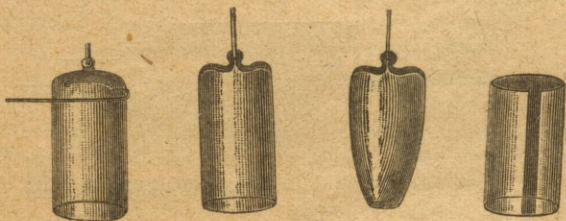
Rys. 38 Kształty szkła podczas wydymania i po przecięciu.
