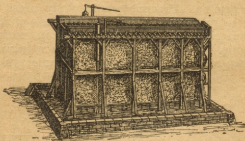
Rys. 35. Tężnia.
