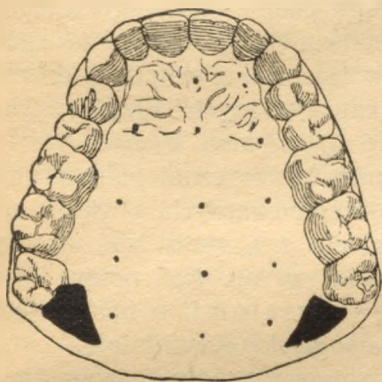
Rys. 59. Samogłoska a w wyrazie pan .
