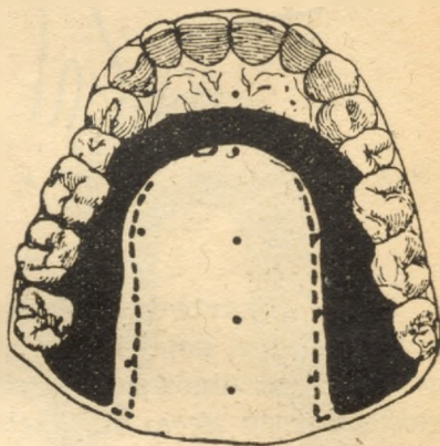
Rys. 46. Miejsce zetknięcia przy ź (plama czarna) i ć (jeszcze po linję przerywaną).
