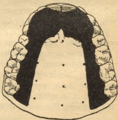
Ryc. 32. Miejsce zetknięcia przy spółgłoskach c w wyrazie co .
