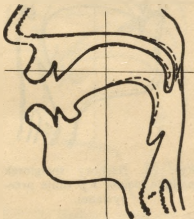
Rys. 22. Połączony obraz nastaw samogłosek õ i o .
