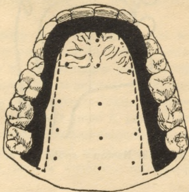
Rys. 28. Miejsce zetknięcia przy spółgłoskach: d , n (miejsce zaczernione) i t (to samo miejsce szersze do linii przerywanej). 1
