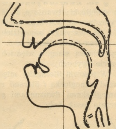
Rys. 20. Połączony obraz nastaw samogłosek ę i e .
