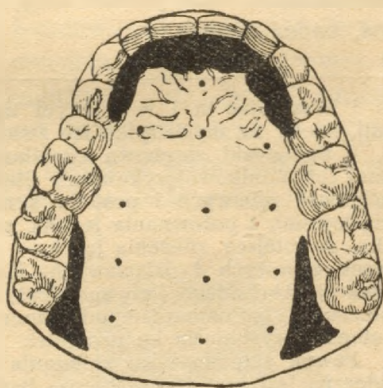
Rys. 34. Miejsce zetknięcia przy spółgłosce ł w wyrazie łuk .
