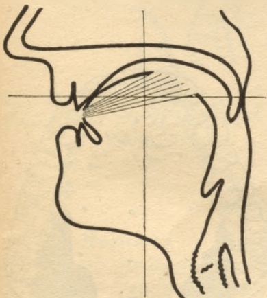
Rys. 50. Nastawy spółgłoski l' .
