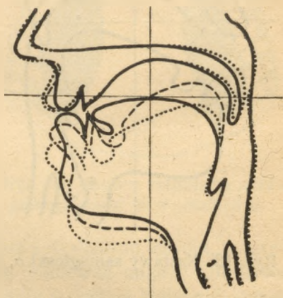
Rys. 18. Połączone obrazy nastaw samogłosek: o — linja kropkowana; u — linja przerywana. Położenie podniebienia miękkiego dla obu samogłosek zaznaczono linją kropkowaną.
