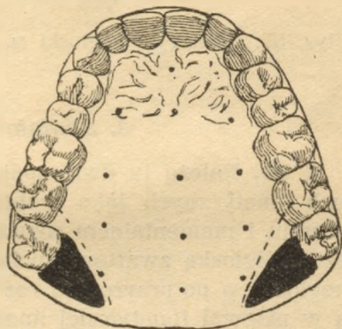
Rys. 56. Miejsce zetknięcia przy \chi w wyrazie ach (plama czarna) i w wyrazie hak (do linji przerywanej).
