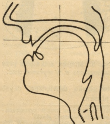
Rys. 11. Nastawy samogłoski i .
