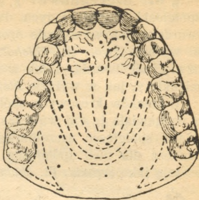
Rys. 58. Miejsce zetknięcia przy n , ń w rozmaitem otoczeniu.
