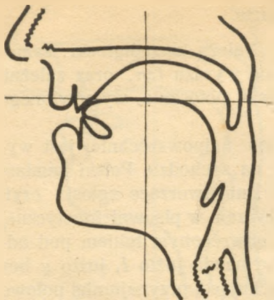
Rys. 35. Nastawy spółgłoski n .
