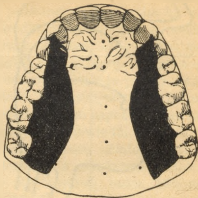
Rys. 10. Miejsce zetknięcia przy samogłosce y w wyrazie my .
