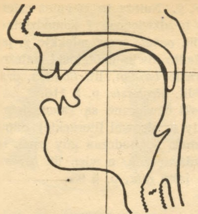
Rys. 57. Nastawy spółgłoski n .
