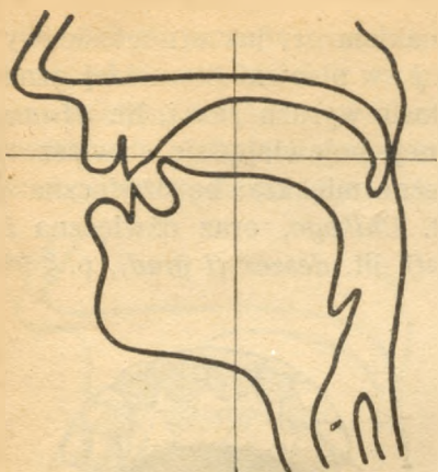
Rys. 42. Nastawy spółgłoski ʃ.
