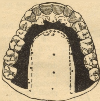
Rys. 44. Miejsce zetknięcia przy d (czarna plama) i t (jeszcze po linię przerywaną).
