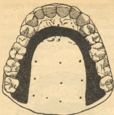
Rys. 52. Miejsce zetknięcia przy n w wyrazie pączek .
