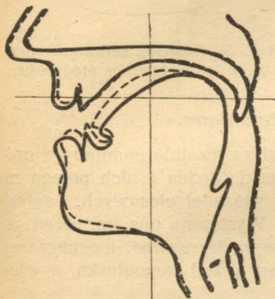
Rys. 55. Nastawy spółgłosek \chi (linja ciągła) i \dot{\chi} (linja przerywana).
