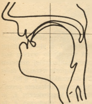
Rys. 38. Nastawy spółgłoski ć.
