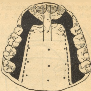
Rys. 30. Miejsce zetknięcia oraz szczeliny przy spółgłoskach: z (plama czarna) i s (po linię przerywaną).
