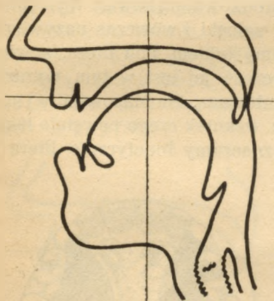
Rys. 7. Nastawy samogłoski e .
