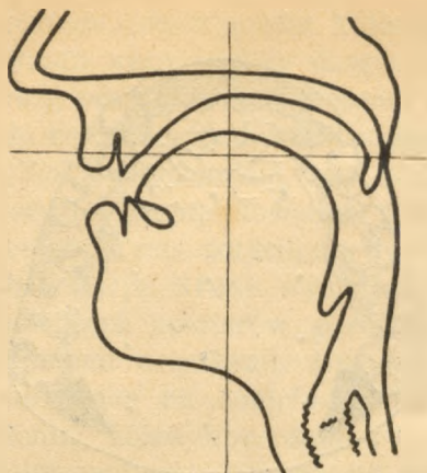
Rys. 9. Nastawy samogłoski y .
