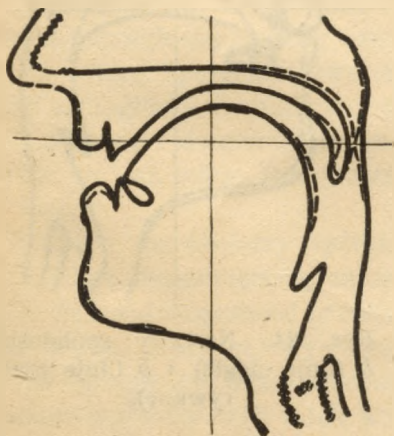
Rys. 21. Połączony obraz nastaw samogłosek ĩ i i .
