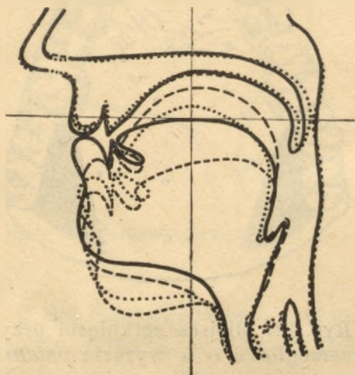
Rys. 17. Połączony obraz nastaw samogłosek: a — linja języka pierwsza od dołu, przerywana, o krótszych odcinkach; e — linja języka środkowa, kropkowana; i — linja języka trzecia od dołu, przerywana o dłuższych odcinkach. Położenie podniebienia miękkiego, zaznaczonego dla wszystkich samogłosek linją kropkowaną.
