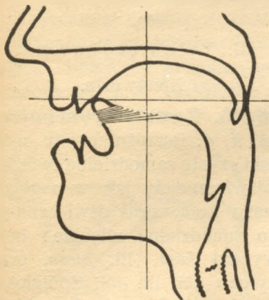
Rys. 48. Nastawy spółgłoski l .
