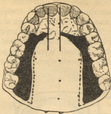
Rys. 43. Miejsce zetknięcia przy ʒ (plama czarna) i ʃ (jeszcze po linię kreskowaną).
