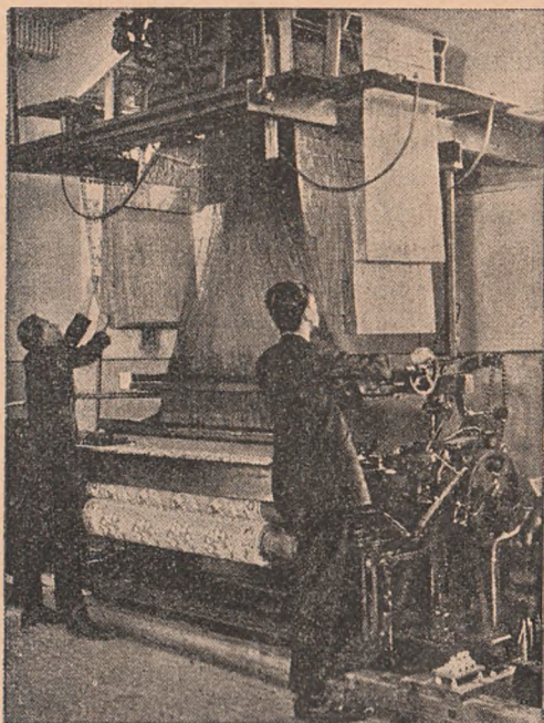
Maszyna systemu Jacquarda
